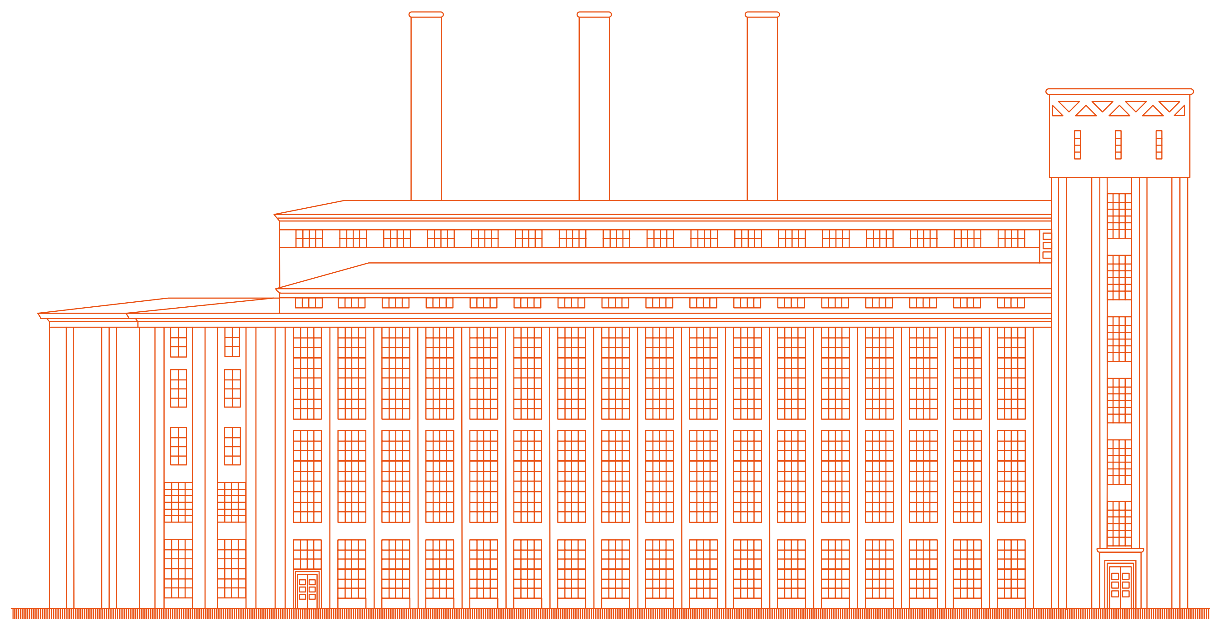
Elektrownia Garbary, elewacja zachodnia, proj. Stefan Cybichowski
